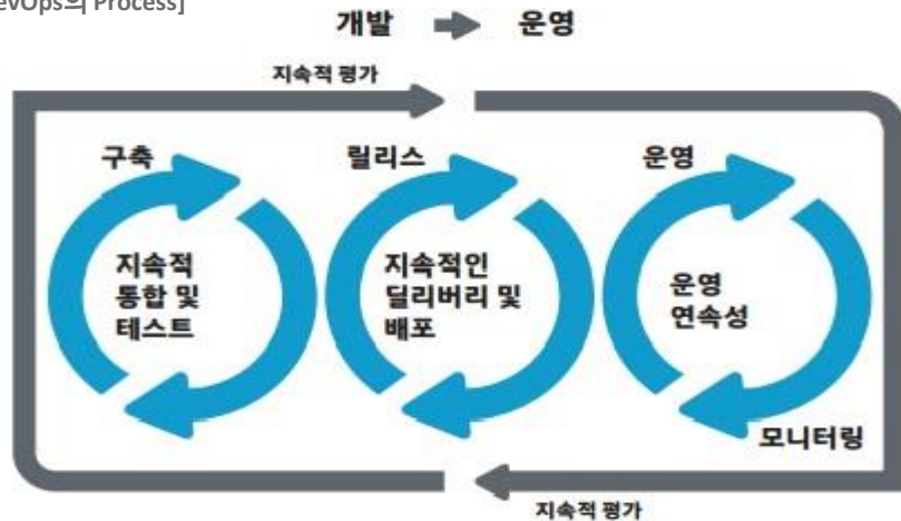
[DevOps의 Process]
